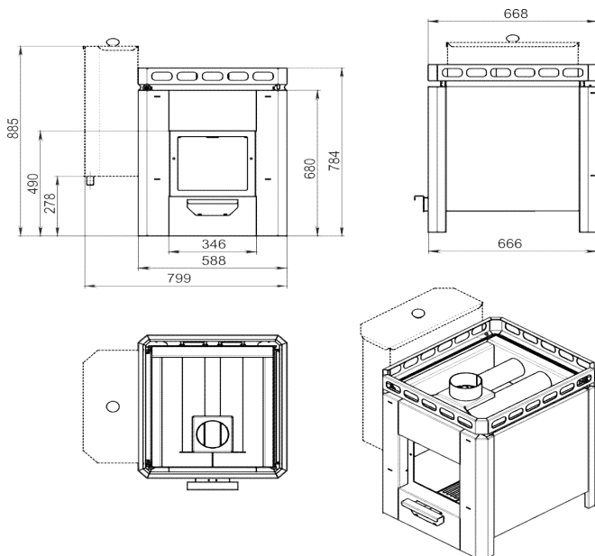
Рисунок 2 – Габаритные размеры печи.
